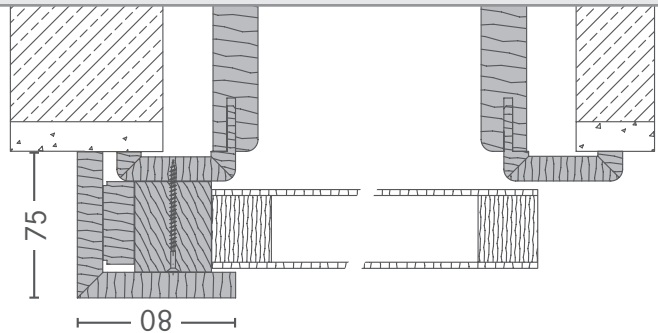
Standard, mit Anschlagpfosten
