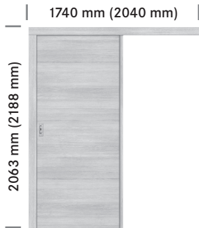
Darstellung von links nach rechts öffnend
