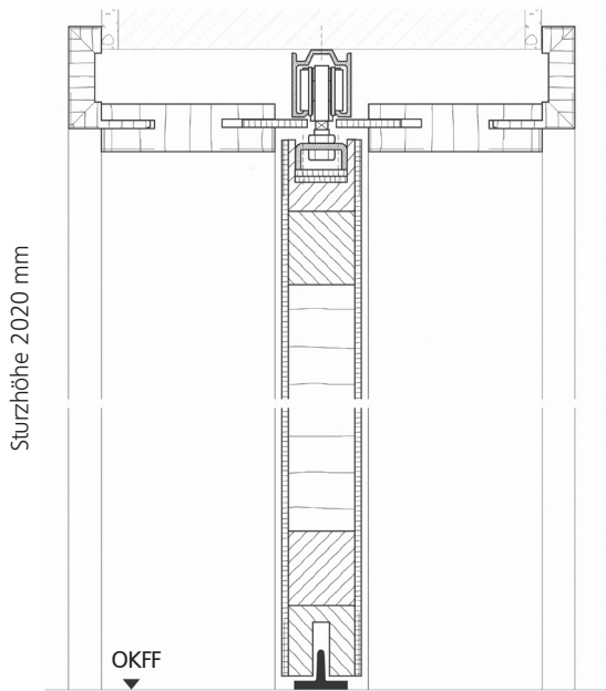
Schiebetür unter Sturz
